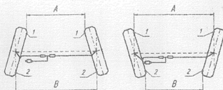
Рисунок 2 - схема измерения схождения передних колес автомобилей
