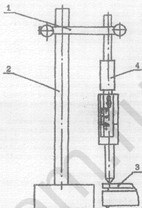
Схема определения измерительного усилия прибора
