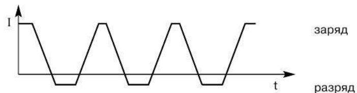
Циклограмма зарядки АКБ в режиме "Реверс".
